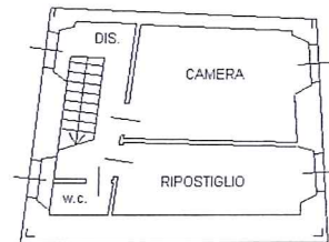
PIANO SECONDO H=235
